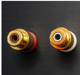
Die Endstufe ist mit ausgezeichneten nextgen-Polklemmen von WBT ausgestattet, Sie ermöglichen den Anschluss eines oder zweier Lautsprecherpaare. Die Polklemmen akzeptieren konfektionierte Kabel mit Bananensteckern oder Kabelschuhen, besitzen jedoch keine Aufnahmen für blanke Litze.
