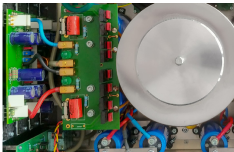
Ein Blick unter die Haube: Hier sehen wir den oberen der beiden übereinander gesetzten Mu-Metall-Transformatoren. Für die Anniversary Edition kommen extrapote Versionen zum Zuge: Jeder dieser Trafos hat eine Lieferfähigkeit von 800 Voltampere - macht in Summe satte 1.600 Voltampere. Am unteren Rand sieht man die kleineren Elkos, die als Pufferung für die großen Elektrolytkondensatoren der Stromversorgung dienen. Ihre Verbindung über Metallschienen sorgt für eine bessere Energieabgabe. Ansonsten verwendet Symphonic Line zur Verbindung extrem hochwertiges Leitermaterial, das auch in den Signalkabeln der Manufaktur zum Einsatz kommt.
