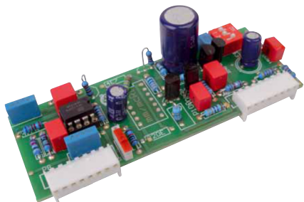
Die eigentliche Phonestufe findet sich direkt am Eingang und kann mit einem Dreifach-DIP-Schalter in ein paar Parametern eingestellt werden
